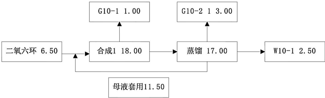
图3.2.10-4 TC-EHS工艺全年二氧六环平衡图 (t/a)
