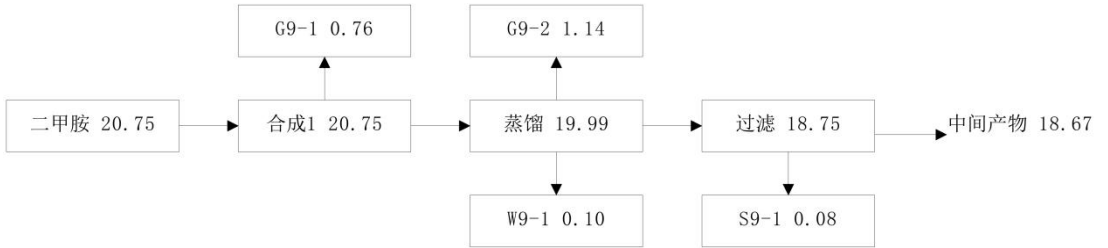
图 3.2.9-4 DPS 工艺全年二甲胺平衡图 (t/a)
