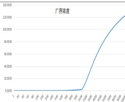
图 5.2.5-10 下游最近厂界处穿透曲线线
