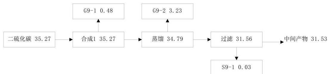
图 3.2.9-5 DPS 工艺全年二硫化碳平衡图 (t/a)
