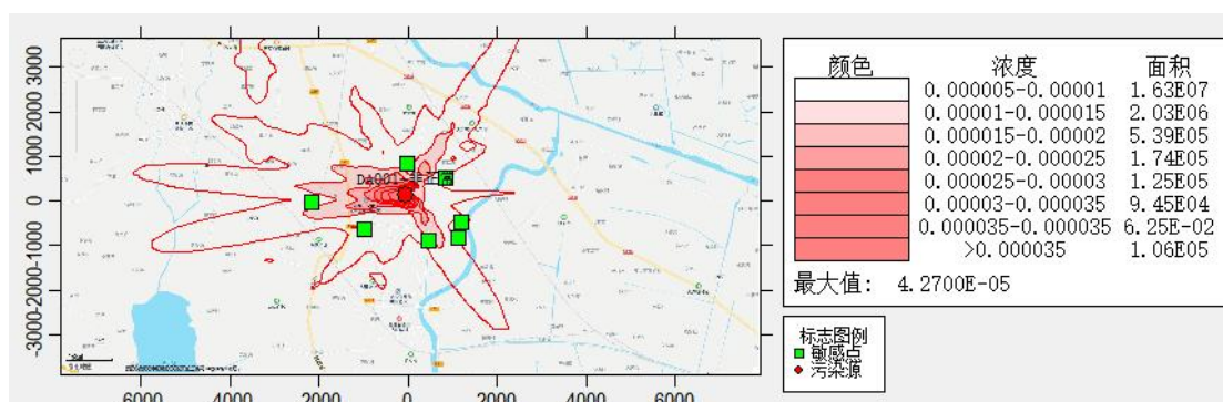
图 5.2-62 非正常排放硫化氢小时值浓度分布图
