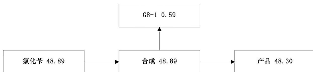
图 3.2.8-4BPC-48 工艺全年氯化苳平衡图 (t/a)
