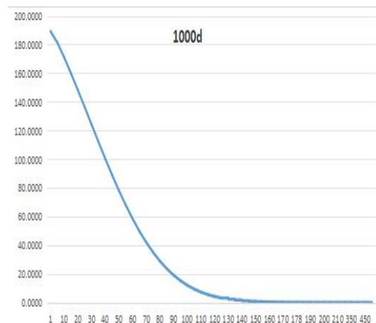
图 5.2.5-8 1000d 污染迁移距离曲线
