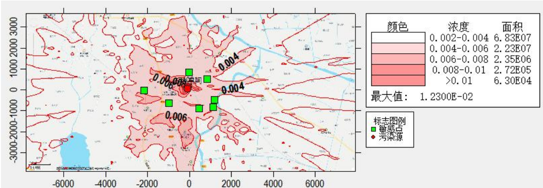
图 5.2-20 PM 2.5 小时值分布图
