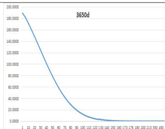
图 5.2.5-9 3650d 污染迁移距离曲线
