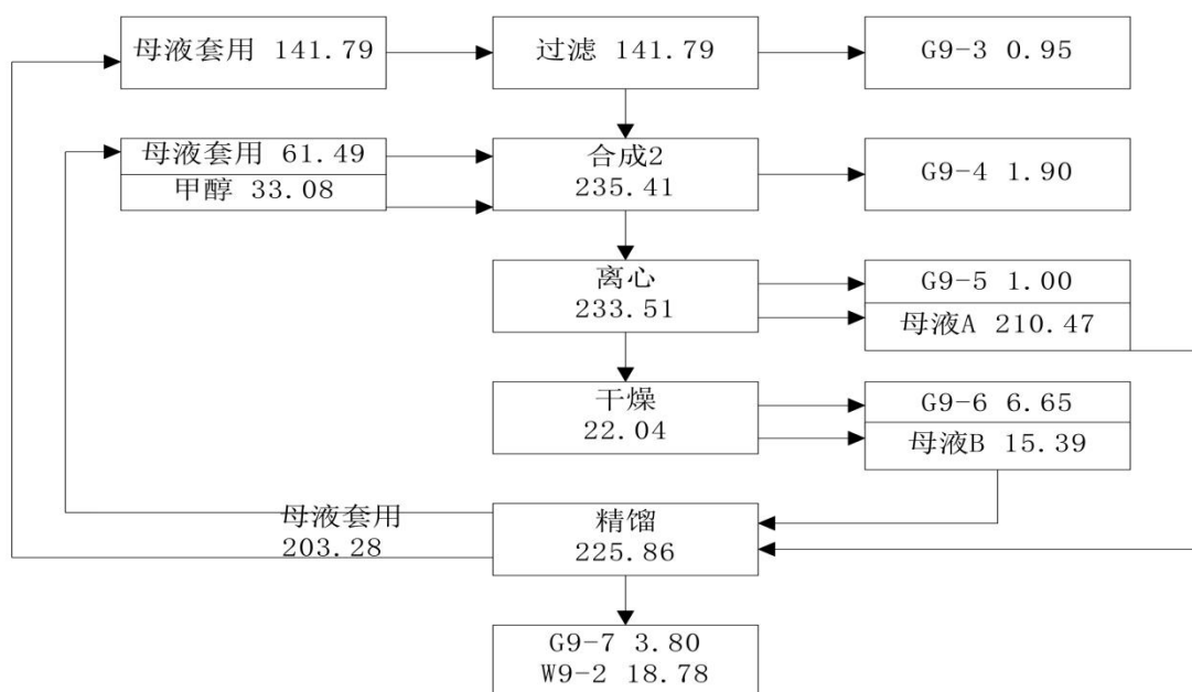
图 3.2.9-6 DPS 工艺全年甲醇平衡图 (t/a)
