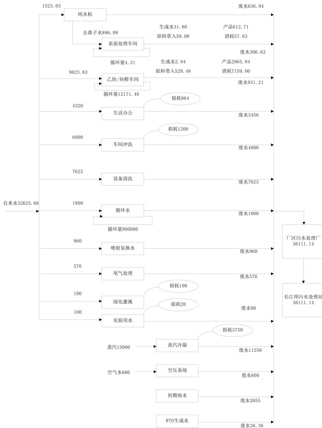
图 3.3.4-1 项目运营期全厂水平衡图 (t/a)
