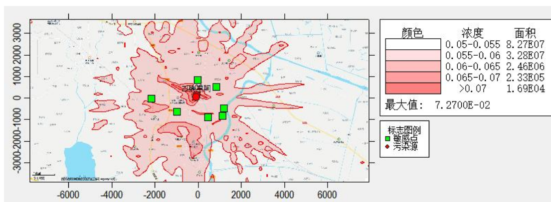
图5.2-39 TSP叠加小时值分布图
