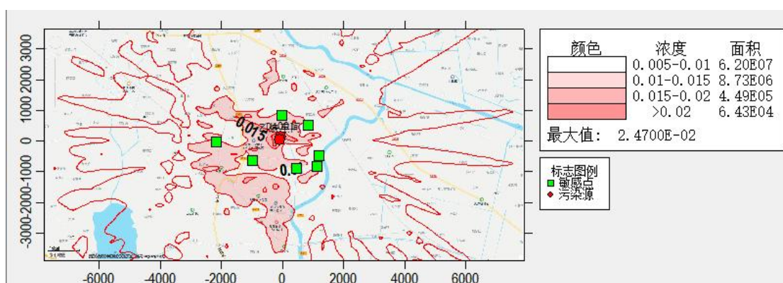
图 5.2-14 TSP 小时值分布图
